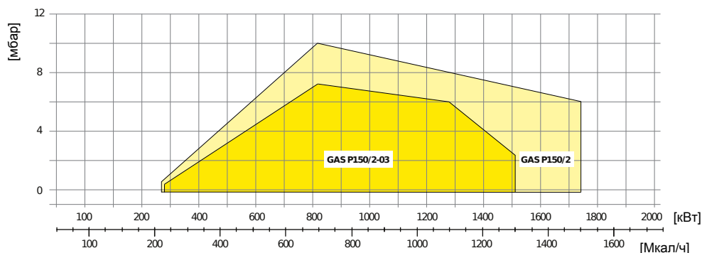
Fig. 2 X = Мощность Y = Сопротивление камеры сгорания
