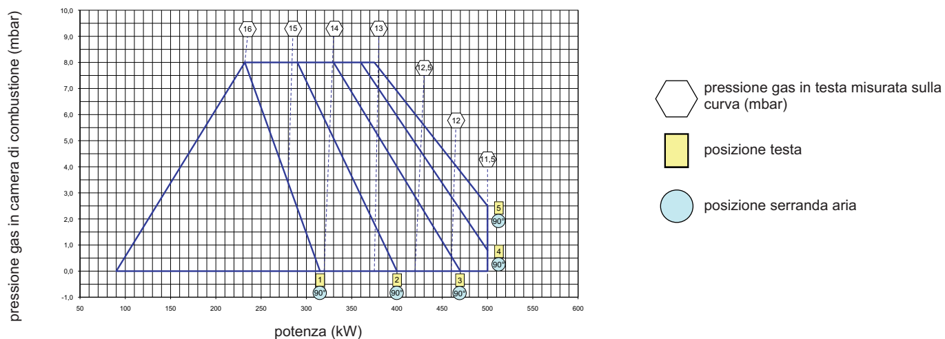
ESEMPIO DI PRETARATURA MAX GAS 500 PAB
